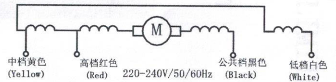
电气原理图 Electrical diagrams
